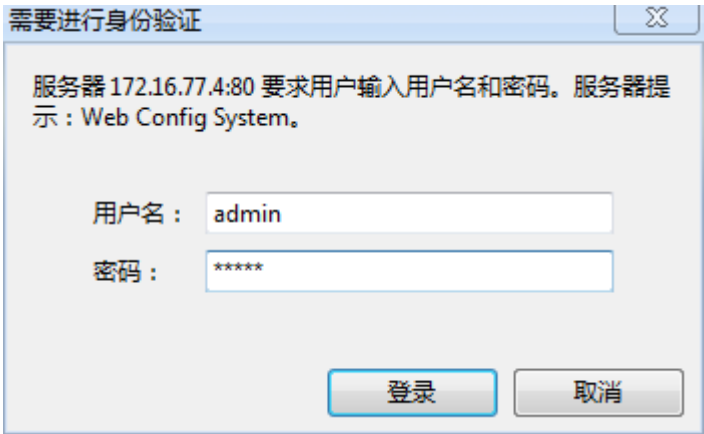
图 4.1-4 登陆界面
